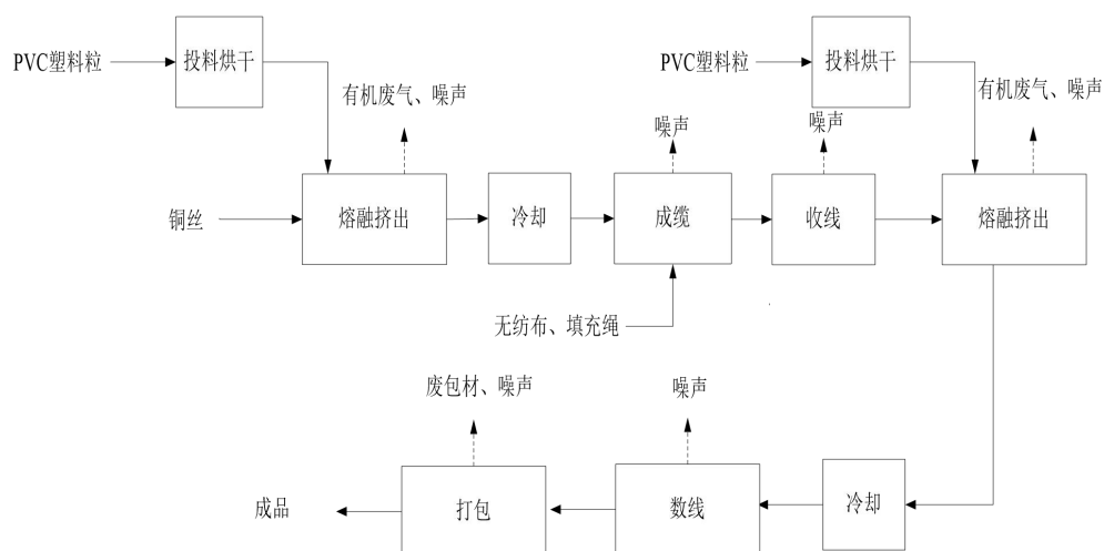
图 2-2 电线电缆生产工艺流程图
