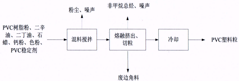
图 2-3 中间品 PVC 塑料粒生产工艺流程图
