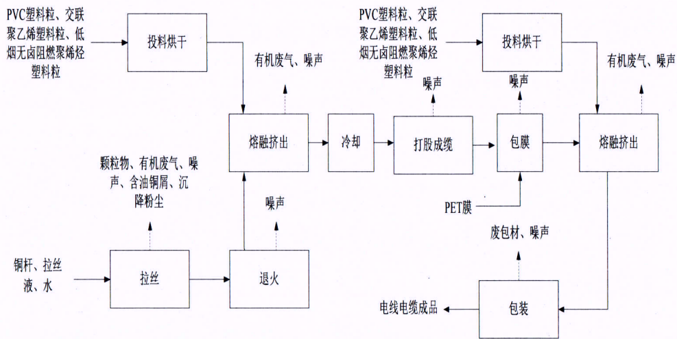
图 2-4 成品生产工艺流程图
