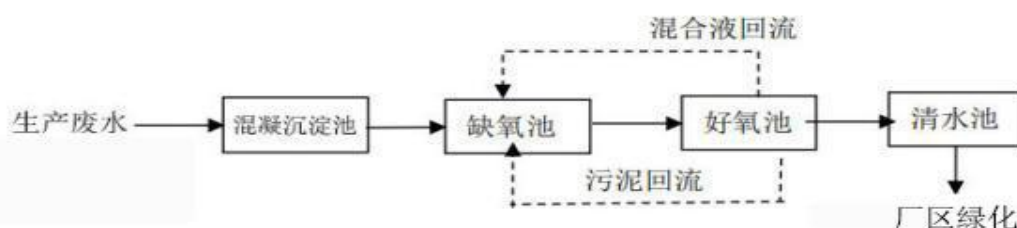
图 4-1 生产废水处理工艺流程图
