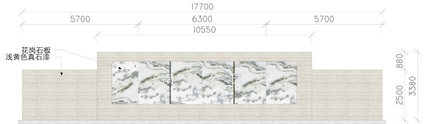
正立面图
