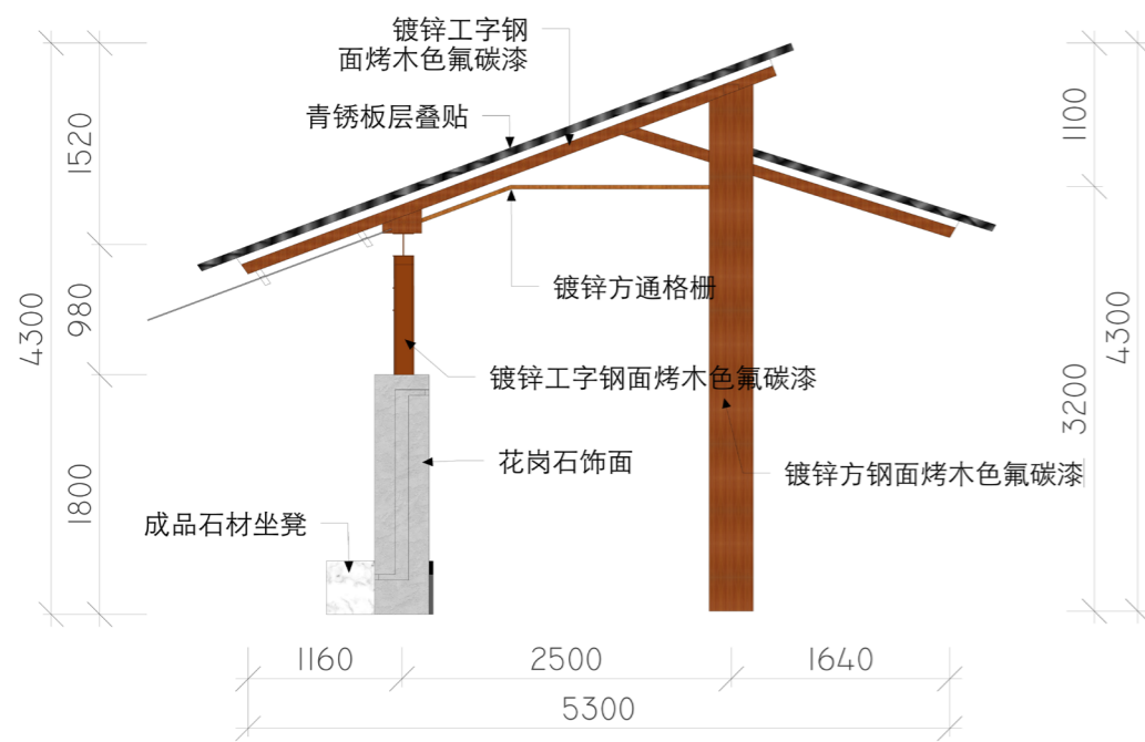
侧立面图
