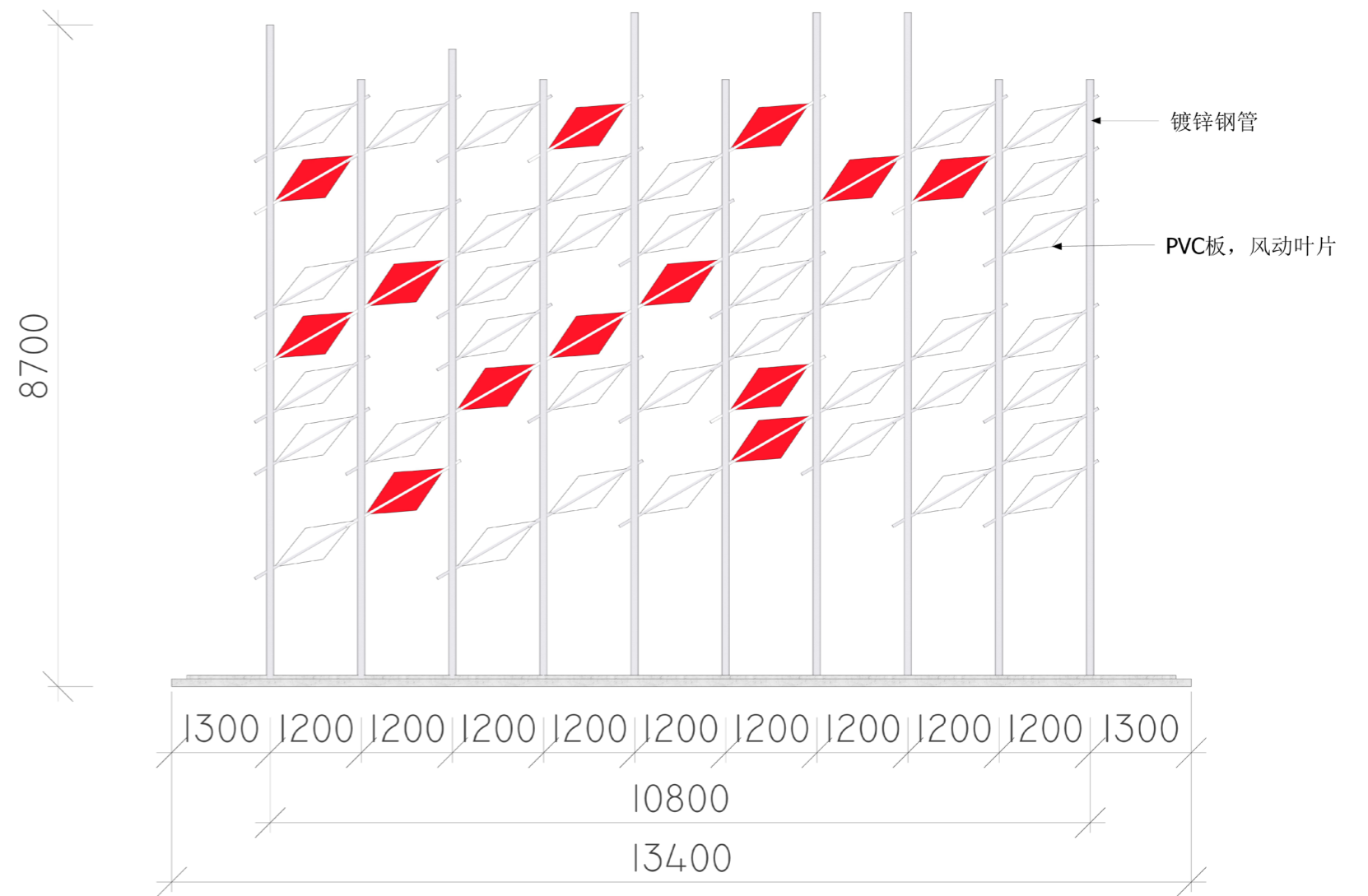
立面图
