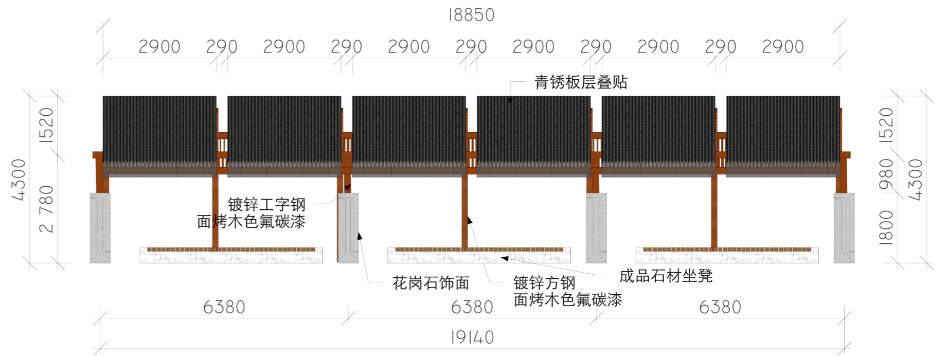
正立面图
