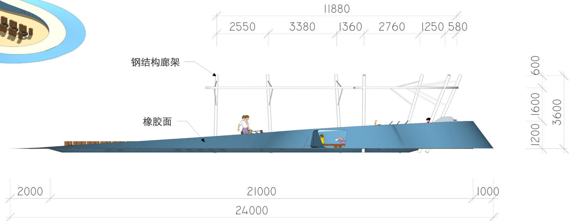
立面图
