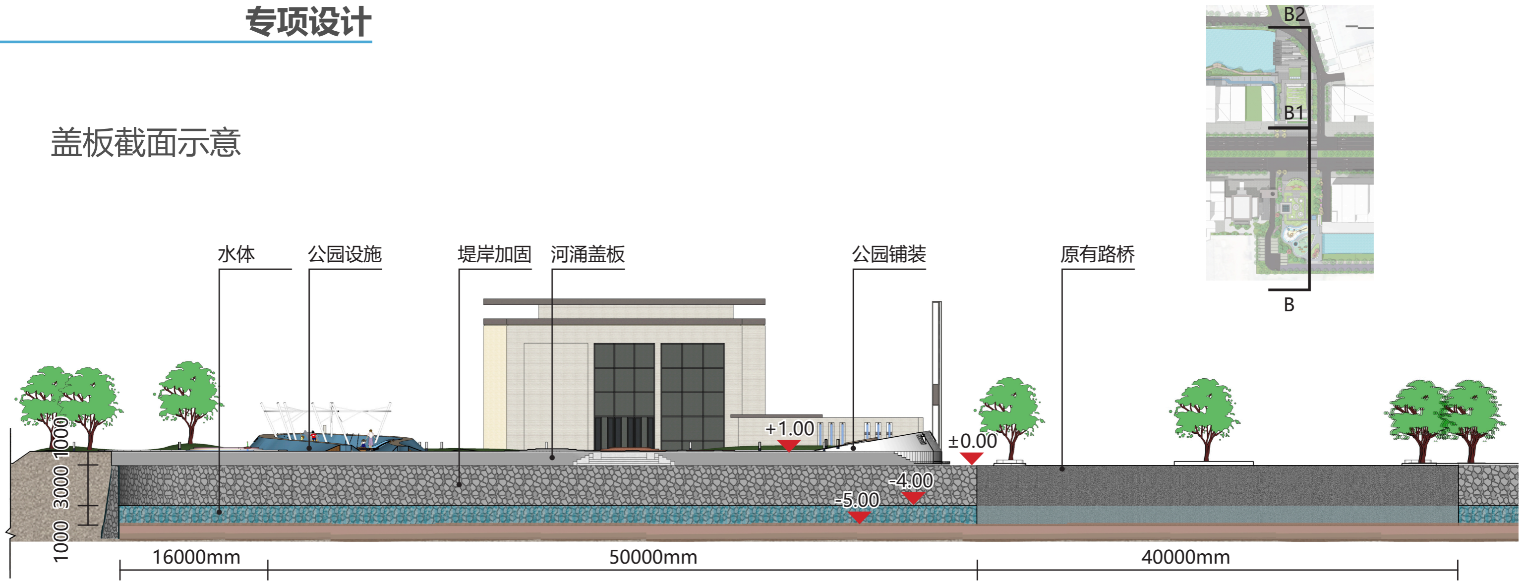
B-B1 剖面图 (具体尺寸以现场实际为准)
