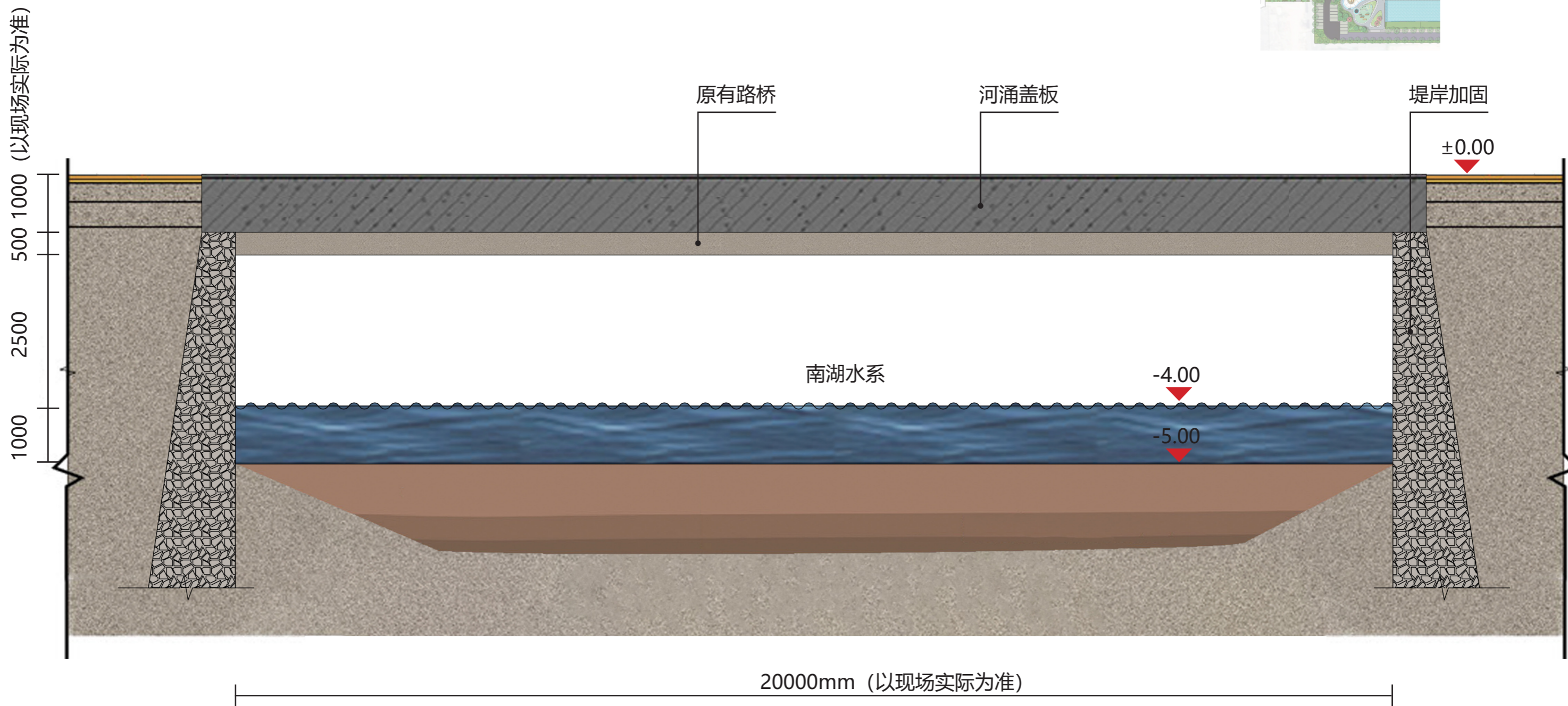
A-A 剖面图
