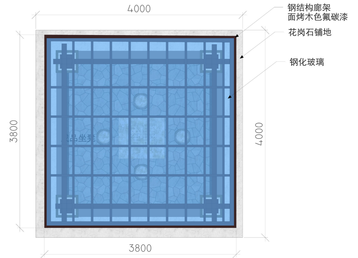
平面图
