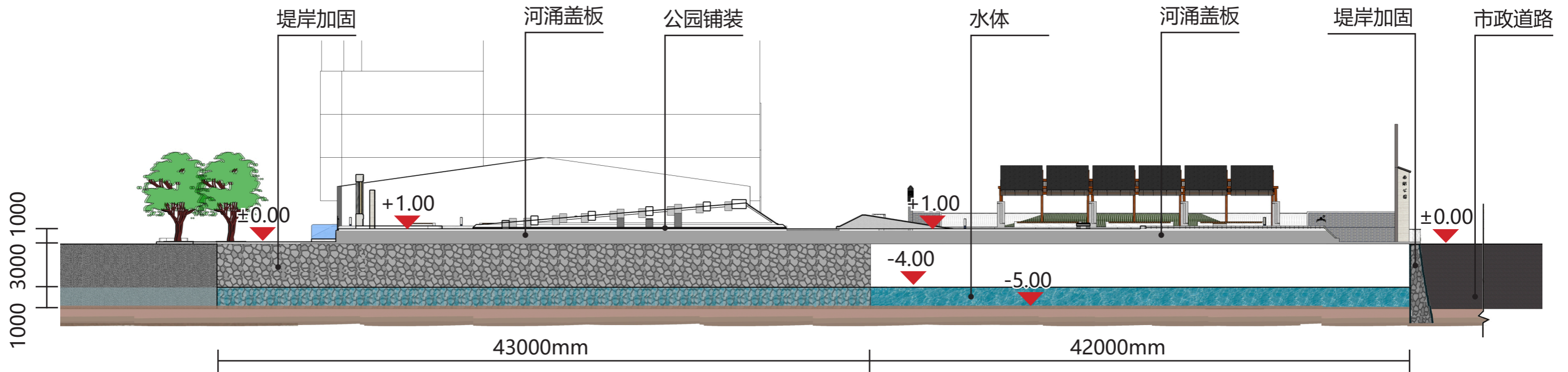
B1-B2 剖面图 (具体尺寸以现场实际为准)
