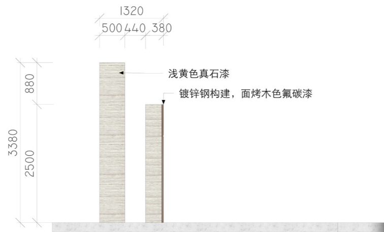
侧立面图
