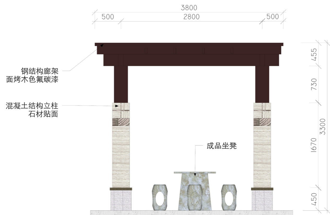
立面图
