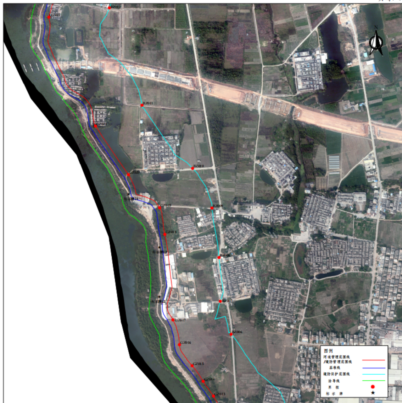
揭西县榕江南河棉湖镇段管理范围与保护范围界线划定图(4/7)
