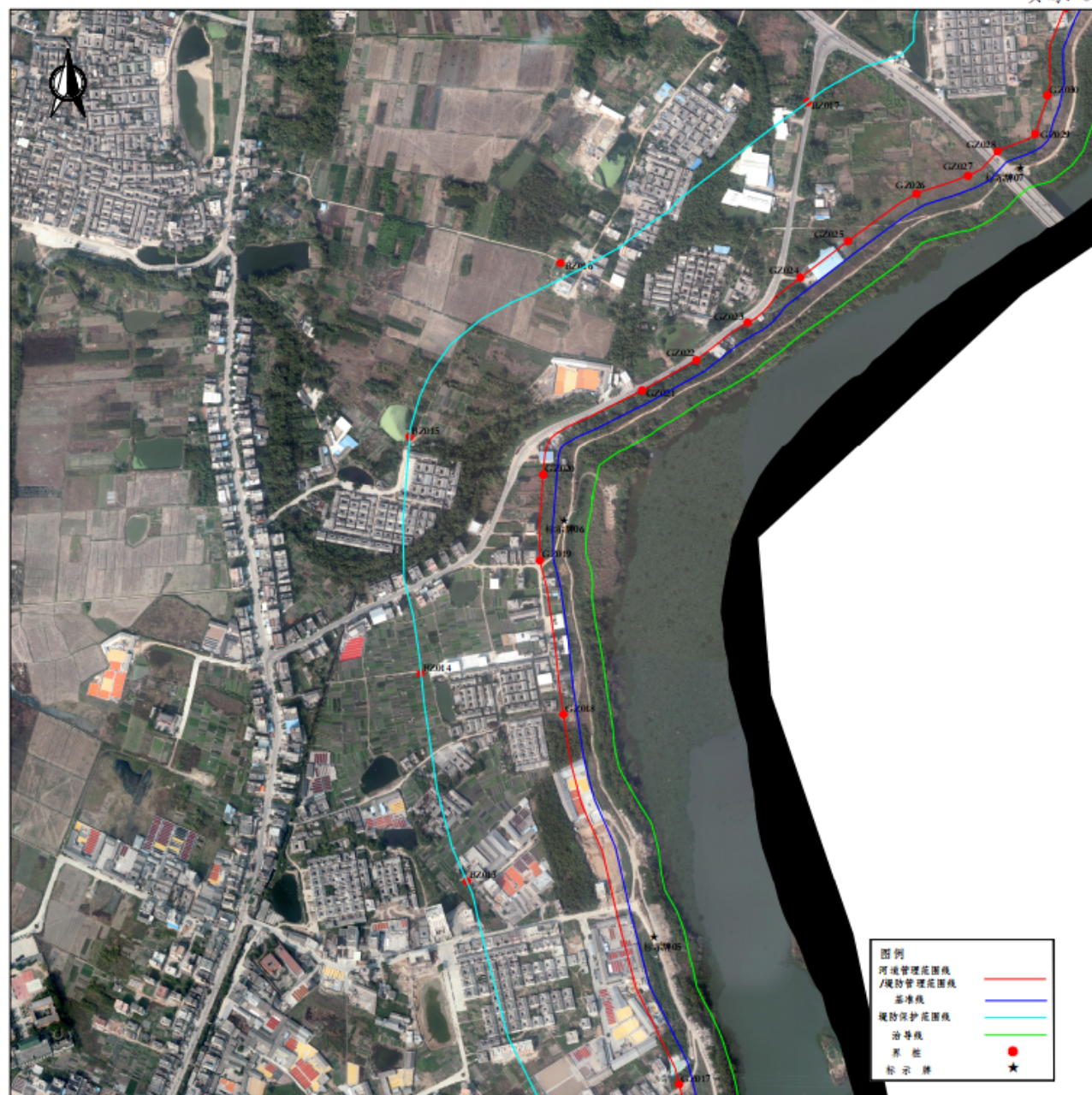
揭西县榕江南河凤江镇段管理范围与保护范围界线划定图(4/7)
