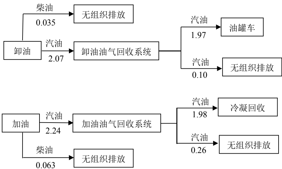
图 7-1 本项目油气平衡图 (t/a)
