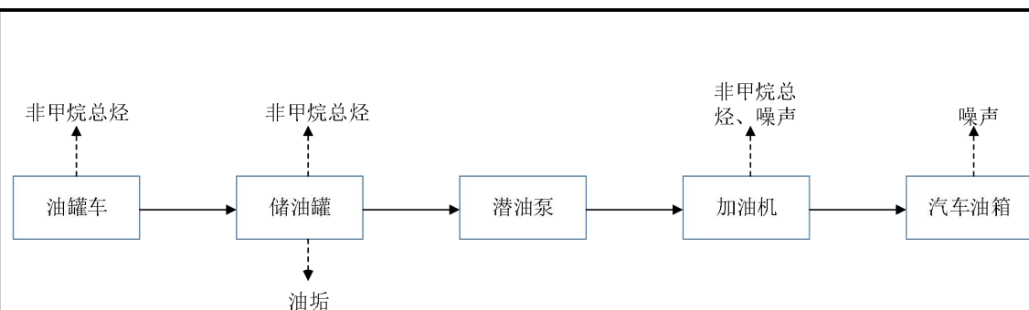
图 5-3 运营期加油（柴油）部分工艺流程及产污节点示意图
