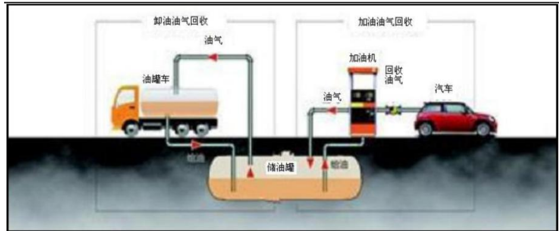
图 5-4 一次、二次油气回收系统示意图
