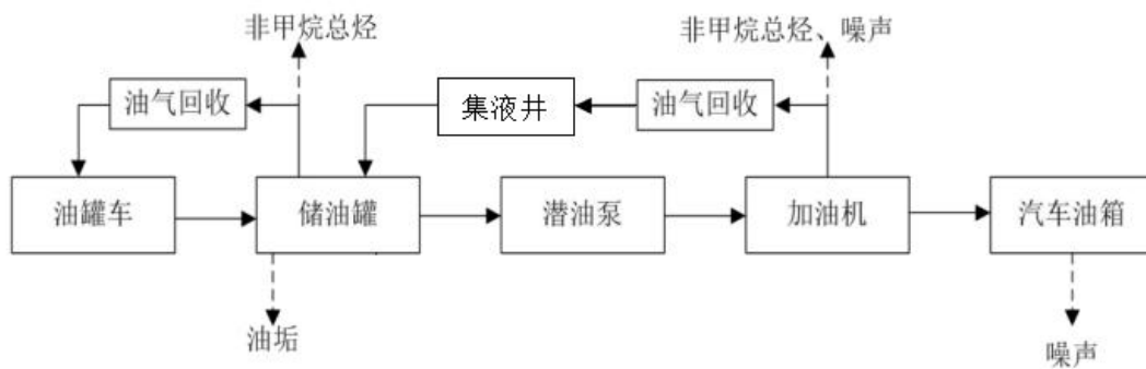
图 5-2 运营期加油（汽油）部分工艺流程及产污节点示意图
