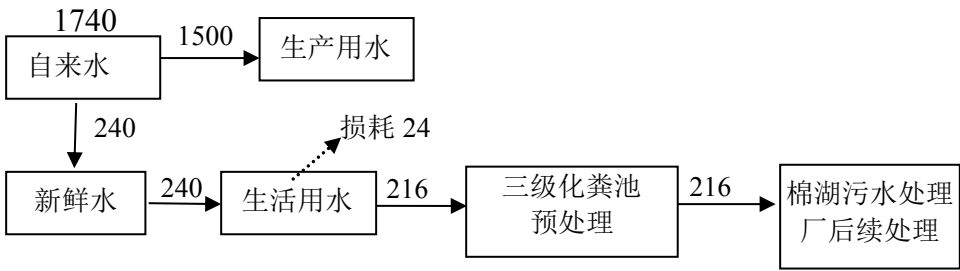
图 1 建设项目水量平衡图（单位：m³/a）
