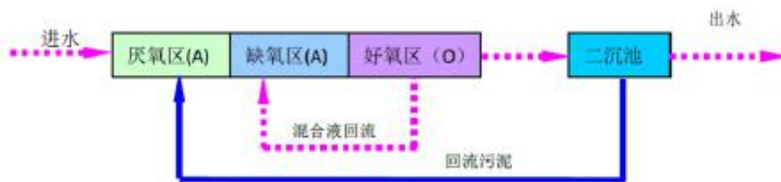
图7-1 传统AAO法工艺流程图
