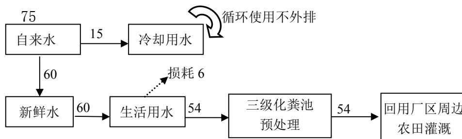
图 1 建设项目水量平衡图 (单位: m 3 /d)
