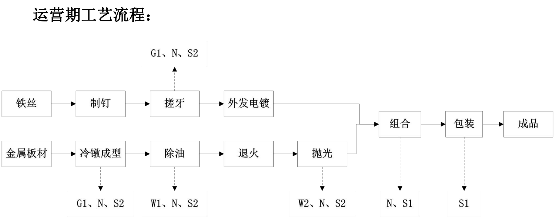
图 5-1 抽芯铆钉生产工艺流程图
