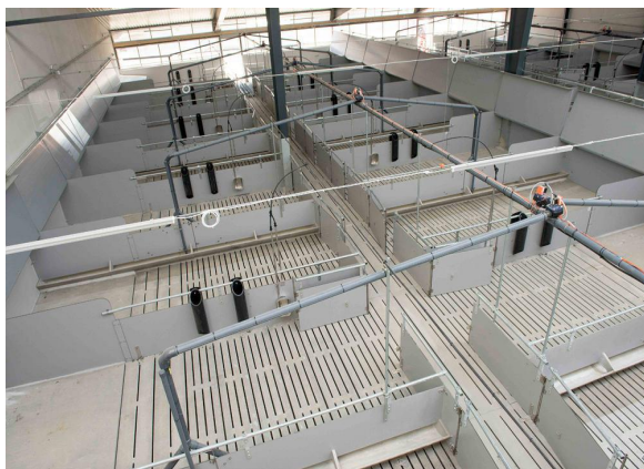
猪舍内部
