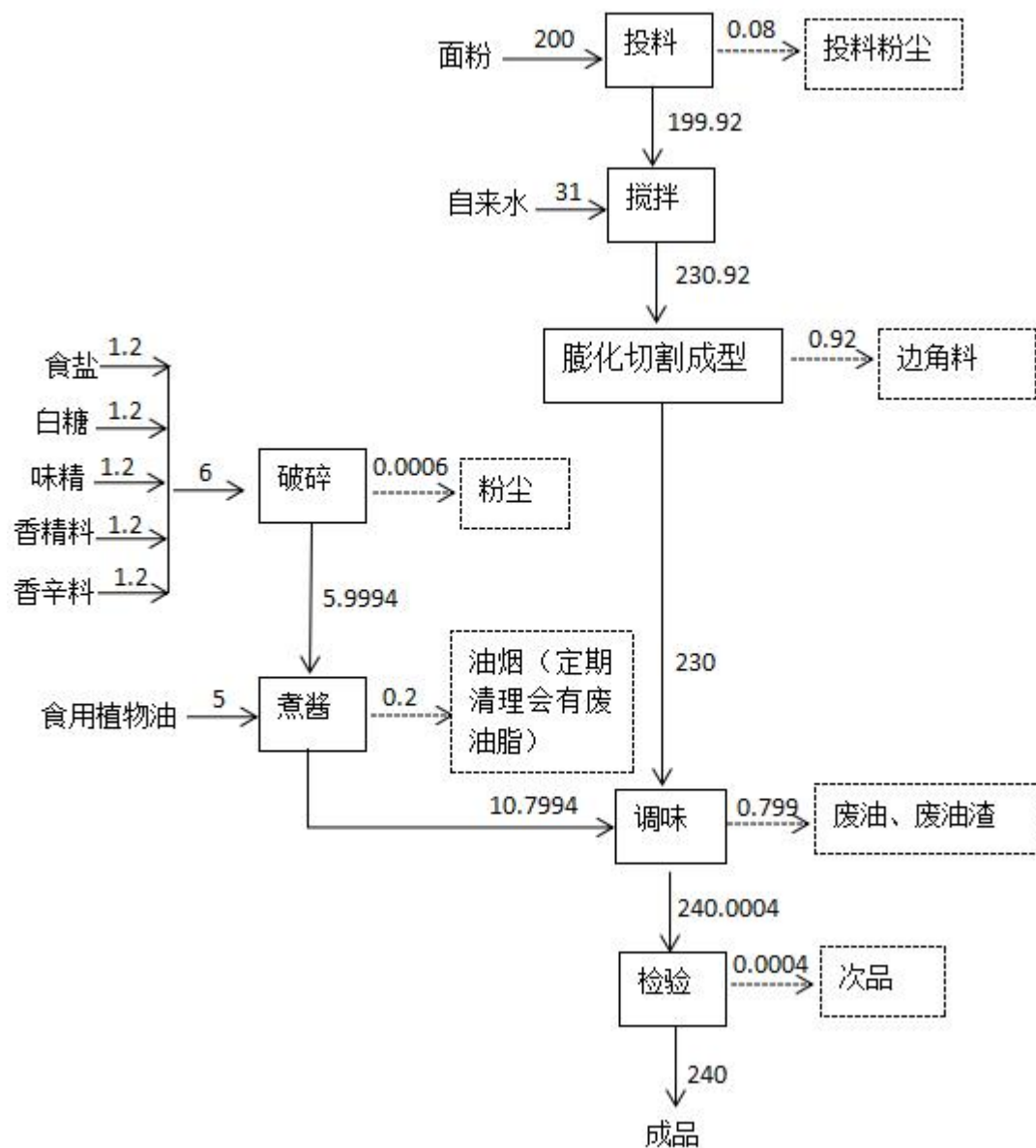
图 4 项目辣条面制食品物料平衡图（单位：t/a）
