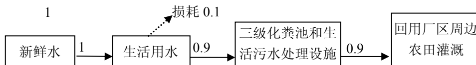
图 1 建设项目水量平衡图（单位：m 3 /d）
