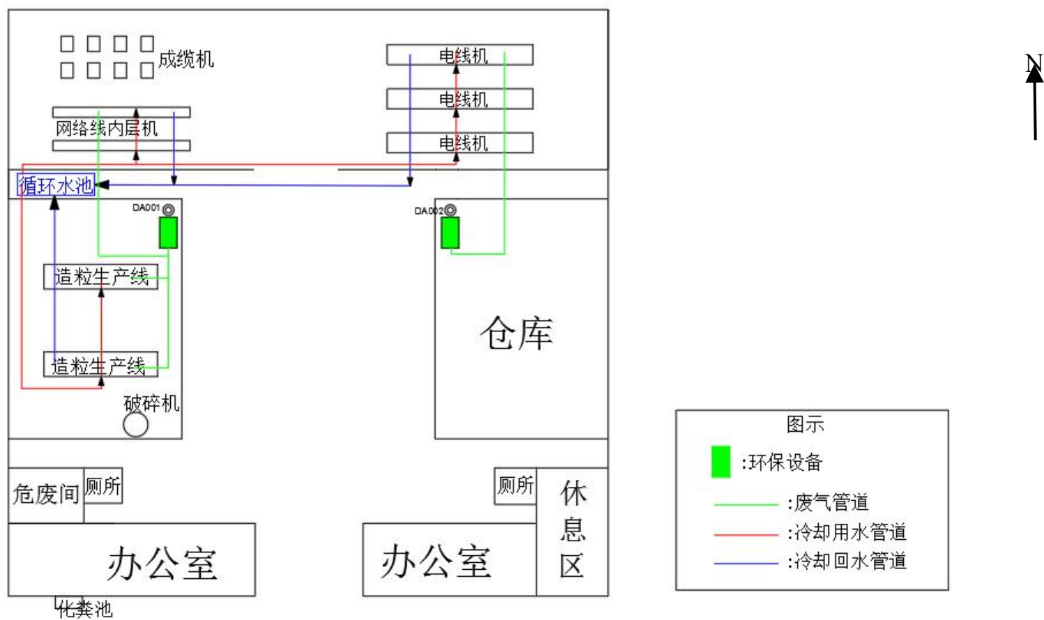
附图 6 项目平面图
