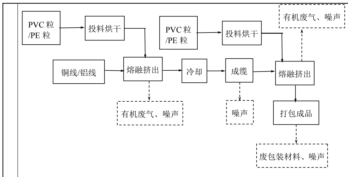
图 2-2 项目电线电缆生产流程及产污图
