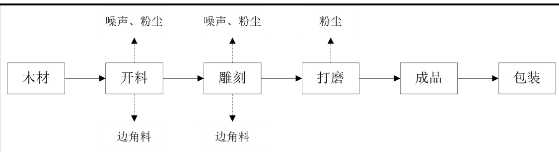
图 1-2 现有项目工艺流程图
