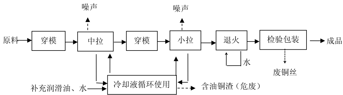
图 1 项目工艺流程及产污环节
