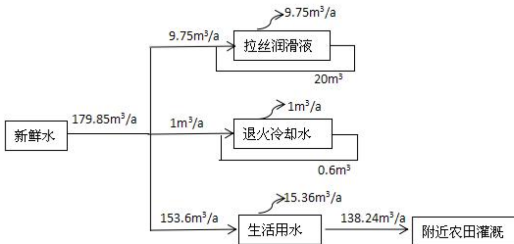
图 2 项目水平衡图
