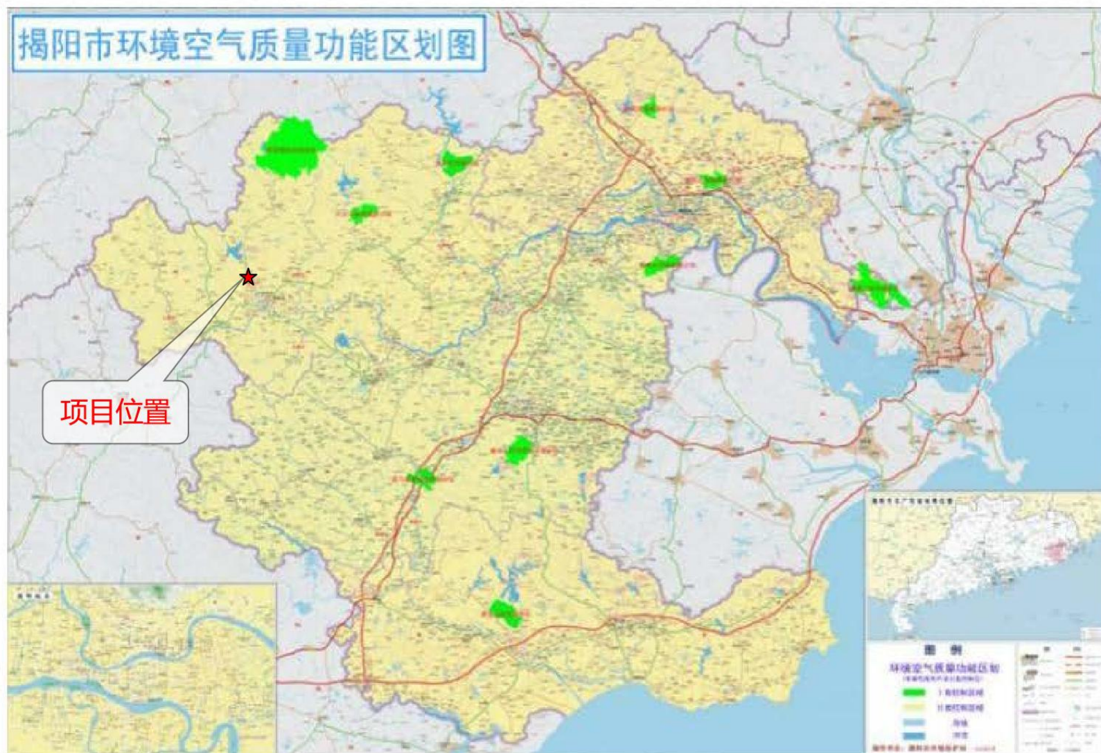
附图 12 揭阳市大气环境功能区划图
