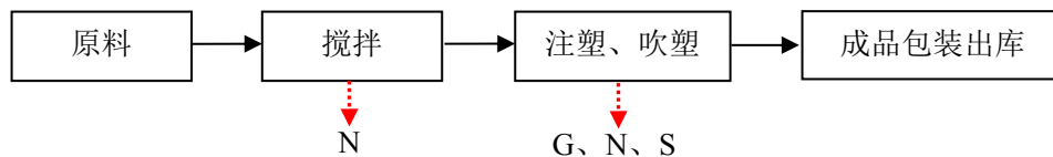
图 4 项目运营期工艺流程图
