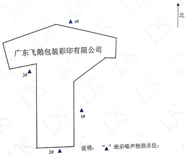
厂界噪声检测点位示意图
