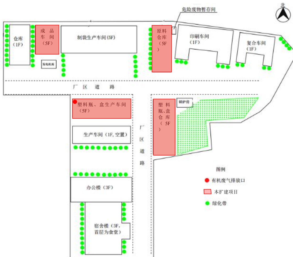
附图 6 项目总平面布局图
