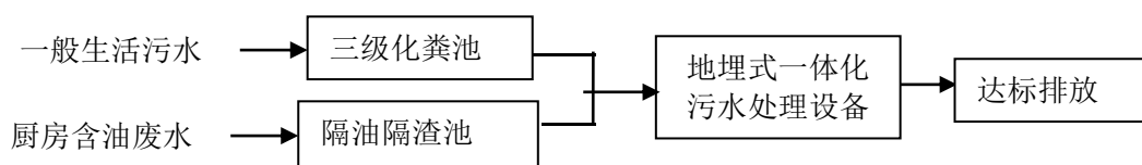
图 5 项目污水处理工艺图
