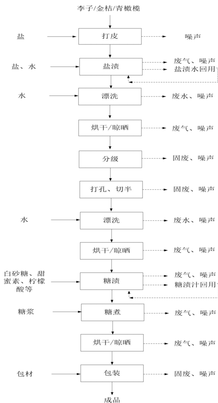
图 2-8 李子、金桔、青橄榄生产工艺流程图
