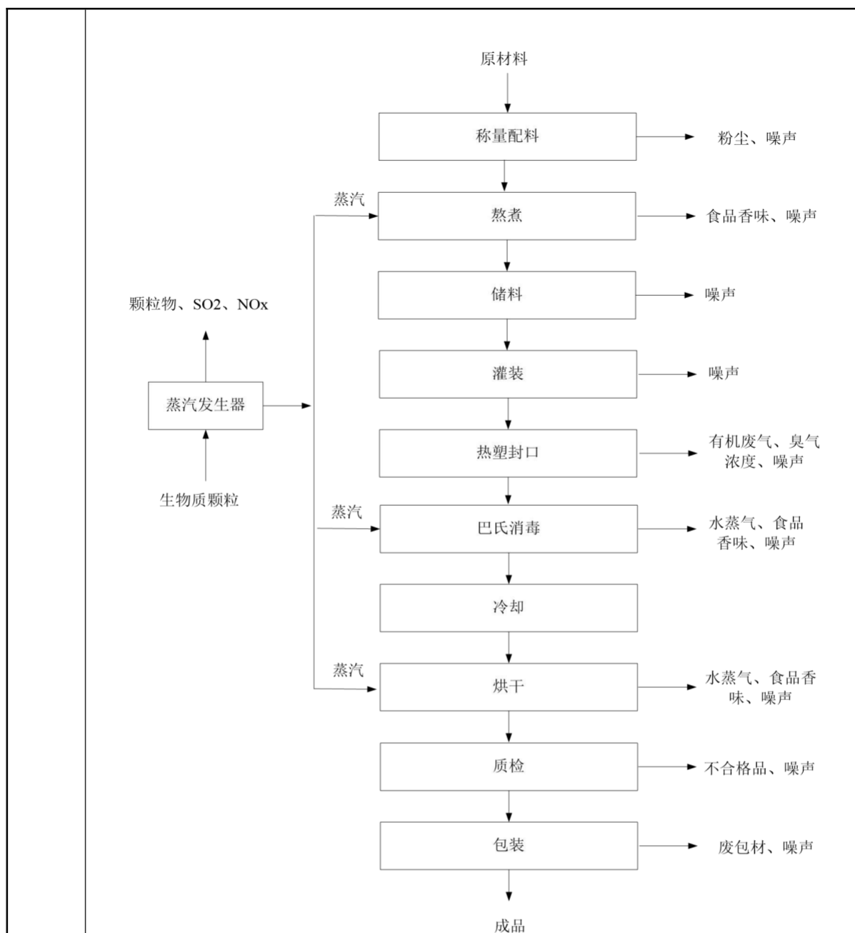
图 2-6 果冻工艺流程图
