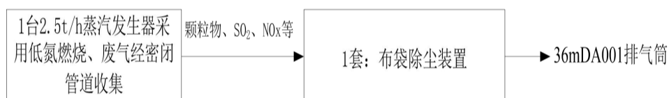
图 4-3 项目蒸汽发生器废气处理工艺流程图
