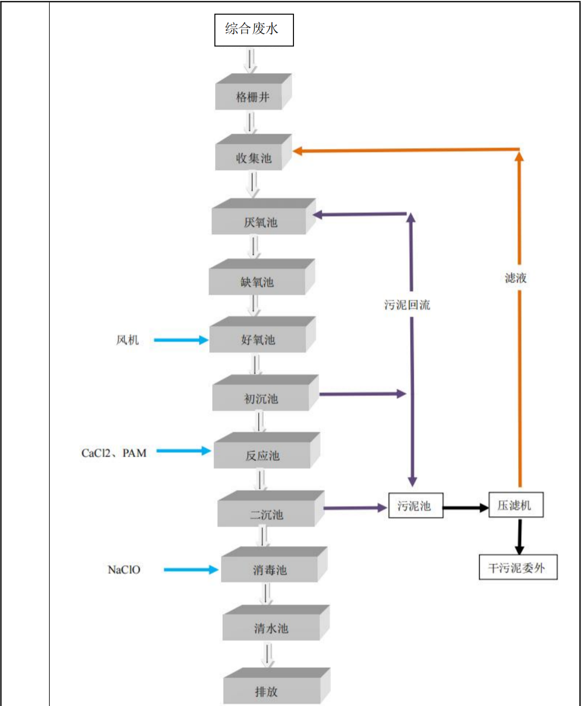
图 4-2 金和镇金鲤开发区污水处理站工艺流程图
