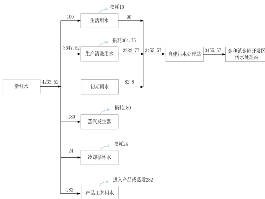
图 2-1 项目用水平衡示意图（单位：t/a）
