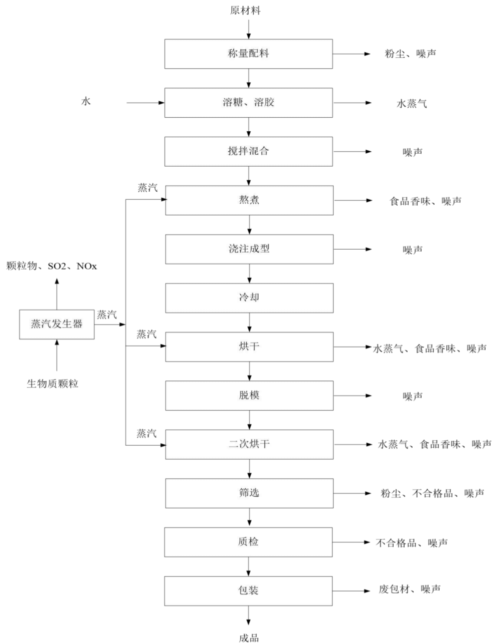
图 2-3 硬糖和软糖工艺流程图
