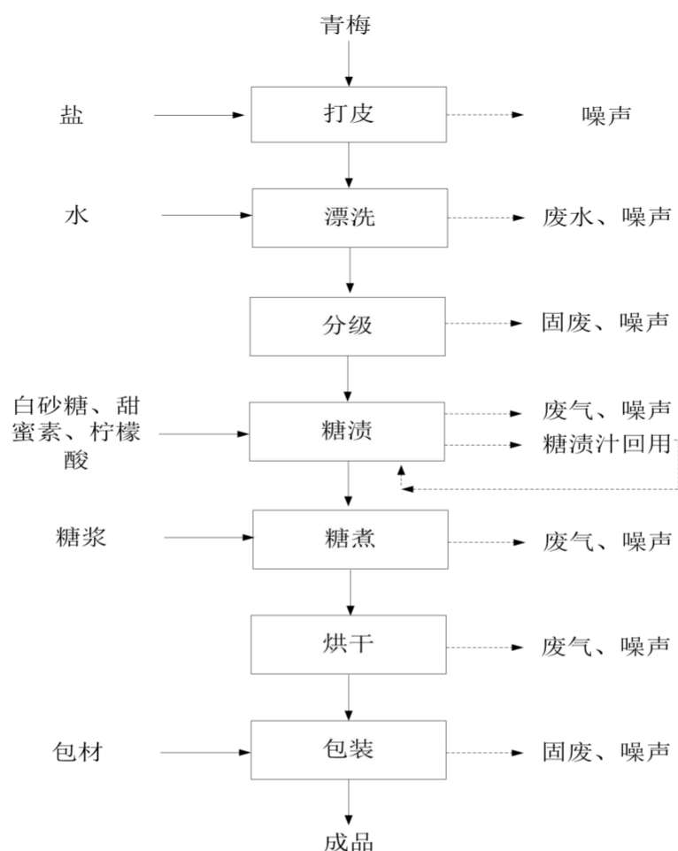
图 2-10 青梅生产工艺流程图
