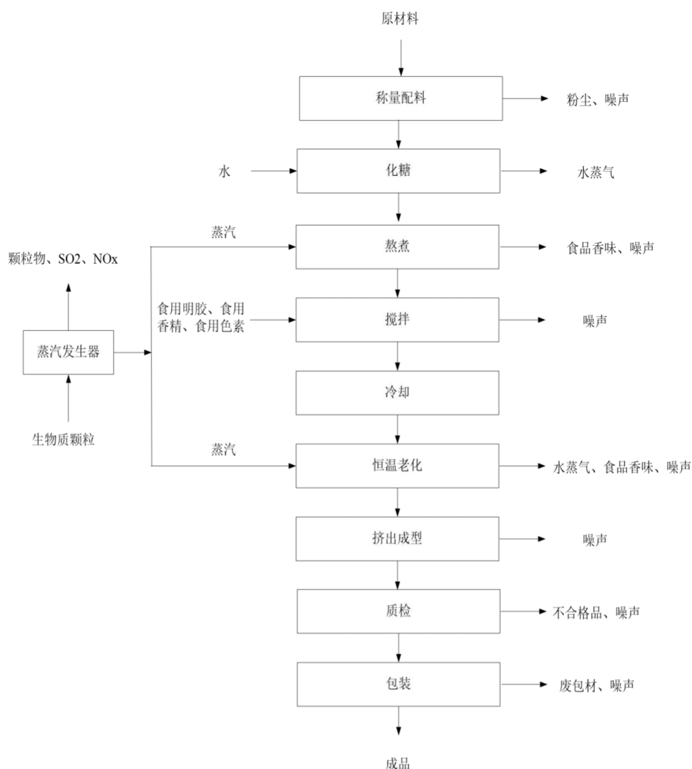
图 2-4 奶糖工艺流程图
