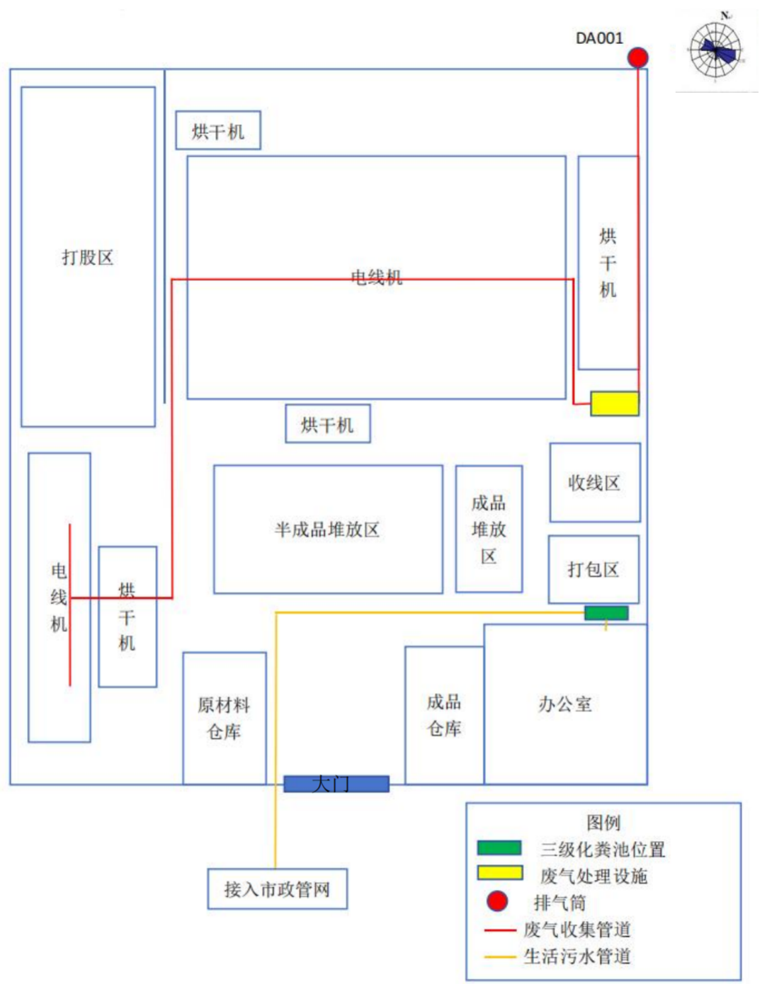
附图 9：平面布局图
