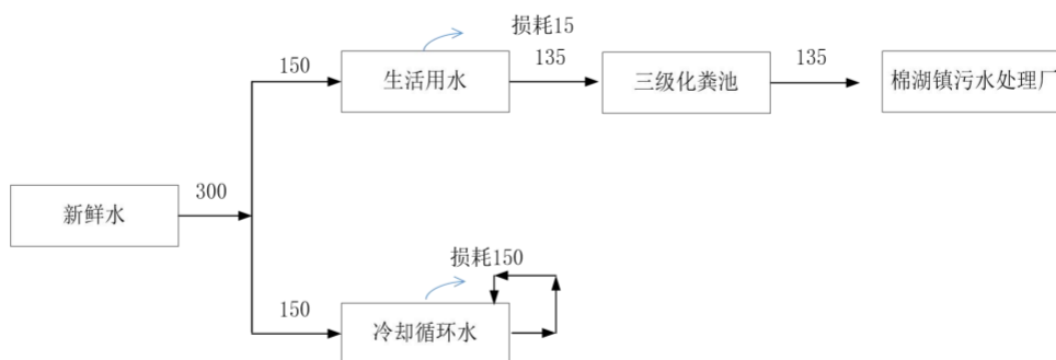
图 2-1 项目用水平衡示意图（单位：t/a）
