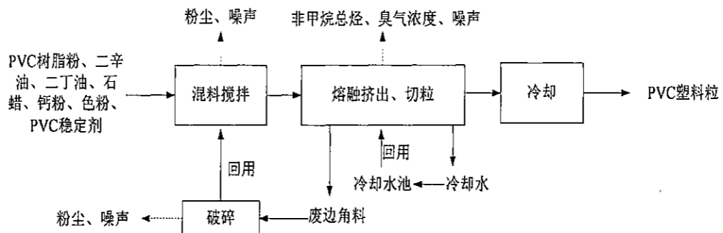
图 2-2 生产工艺流程及产污节点图
