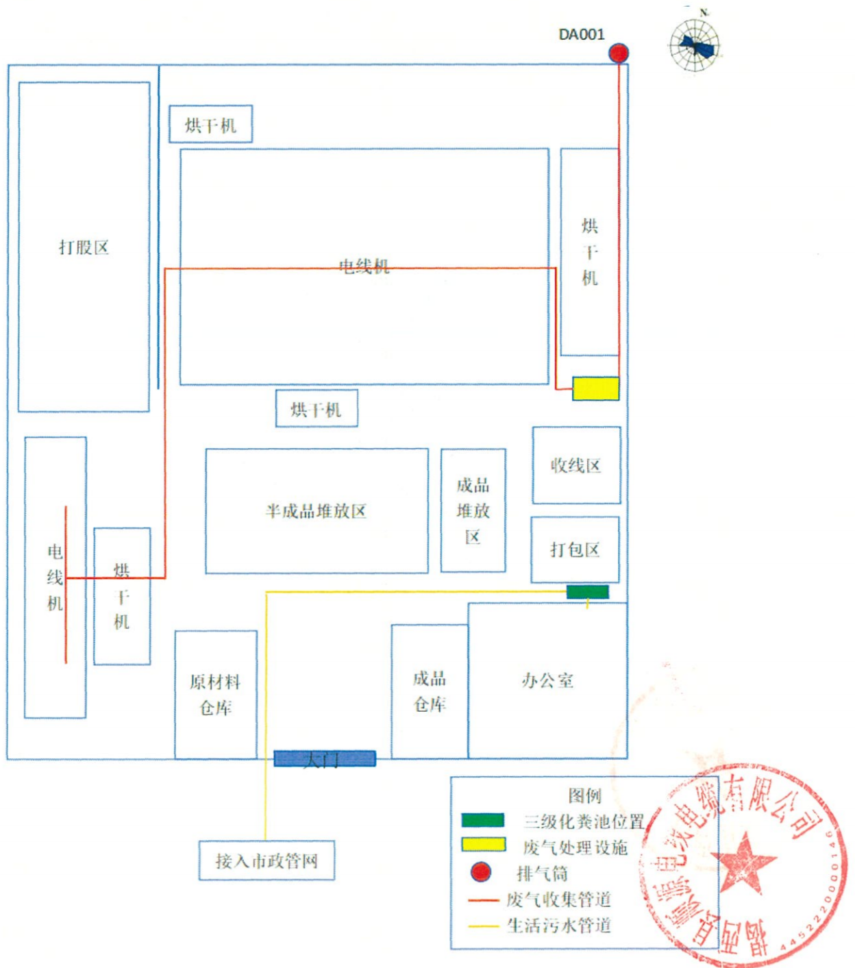
附图 9：平面布局图
