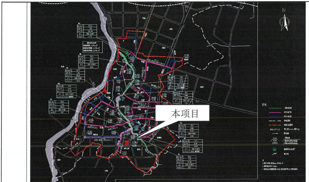
图 4-2 棉湖镇污水处理厂纳污范围图
