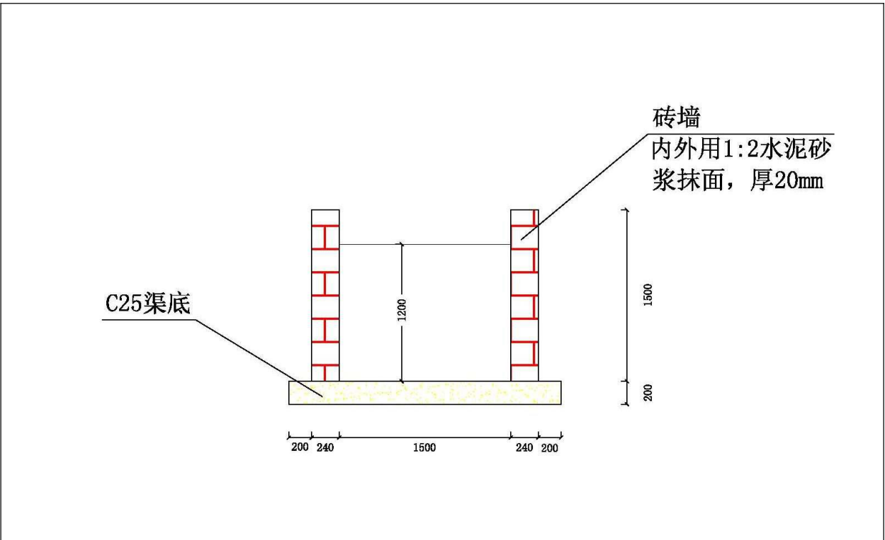
图 1-6 排洪渠改造断面示意图
