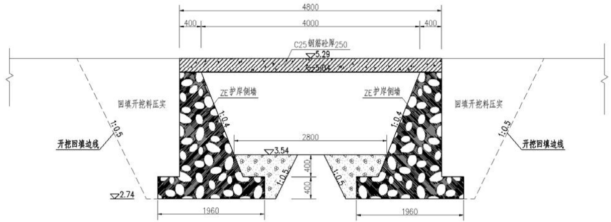
图 2 农桥设计断面示意图
