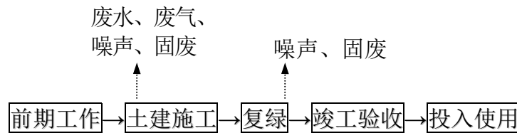
图 6 项目堤防、护岸、农桥、水陂、箱涵、涵洞施工流程图
