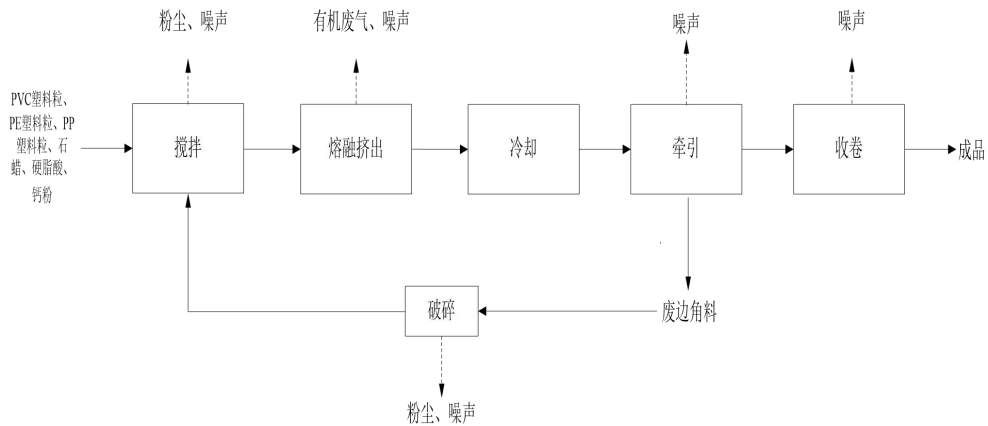
图 2-3 填充绳、绕包带生产工艺流程图
