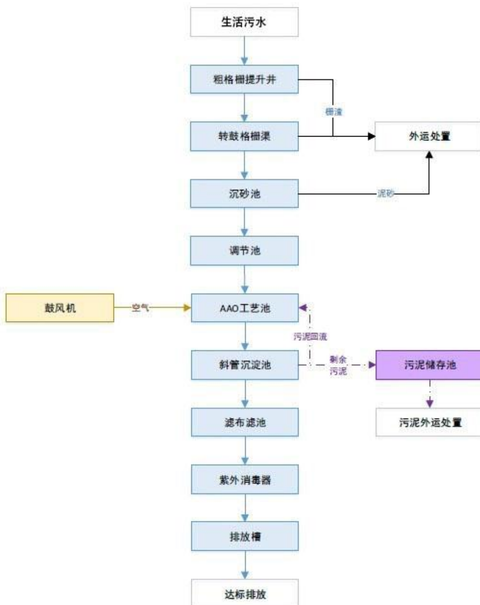
图 5-2 污水处理厂处理工艺流程图
