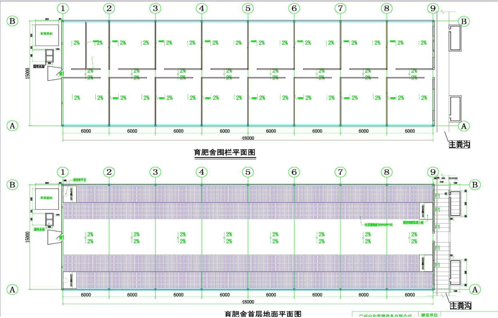
附图 3 育肥舍围栏平面图
