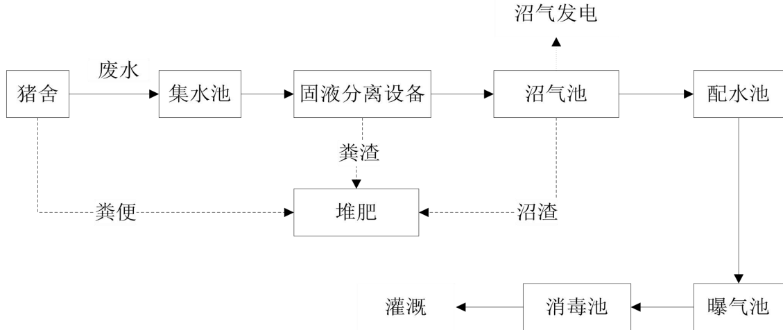
图 7.2-1 废水处理工艺流程
