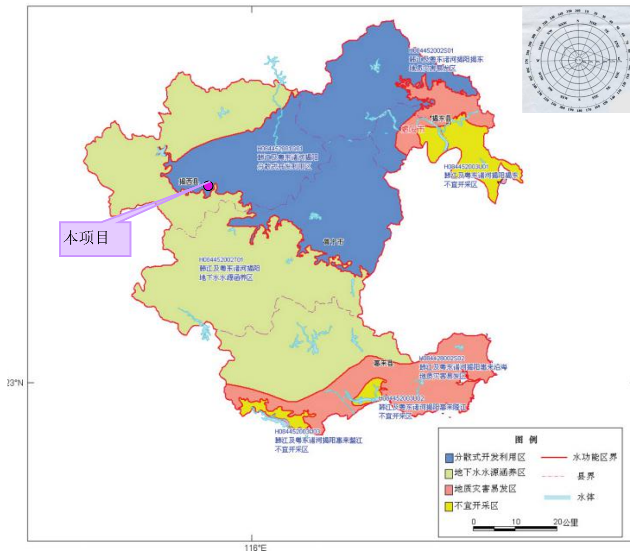
图 1.3-3 揭阳市浅层地下水环境功能区划图
