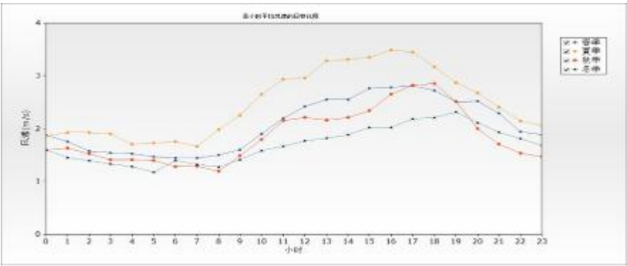
图 6.1-4 各季小时月平均风速变化曲线
