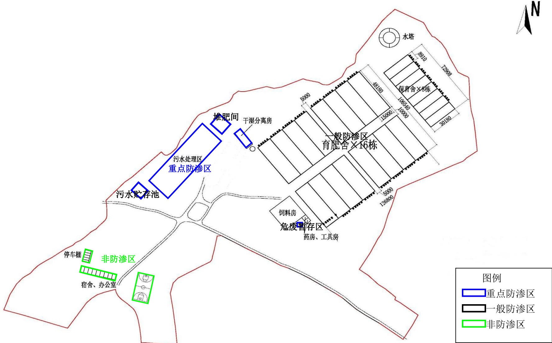
图 7.2-2 项目地下水分区防渗图
