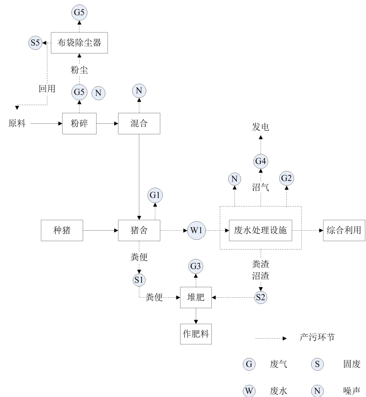
图 3.2-2 项目产污环节图
