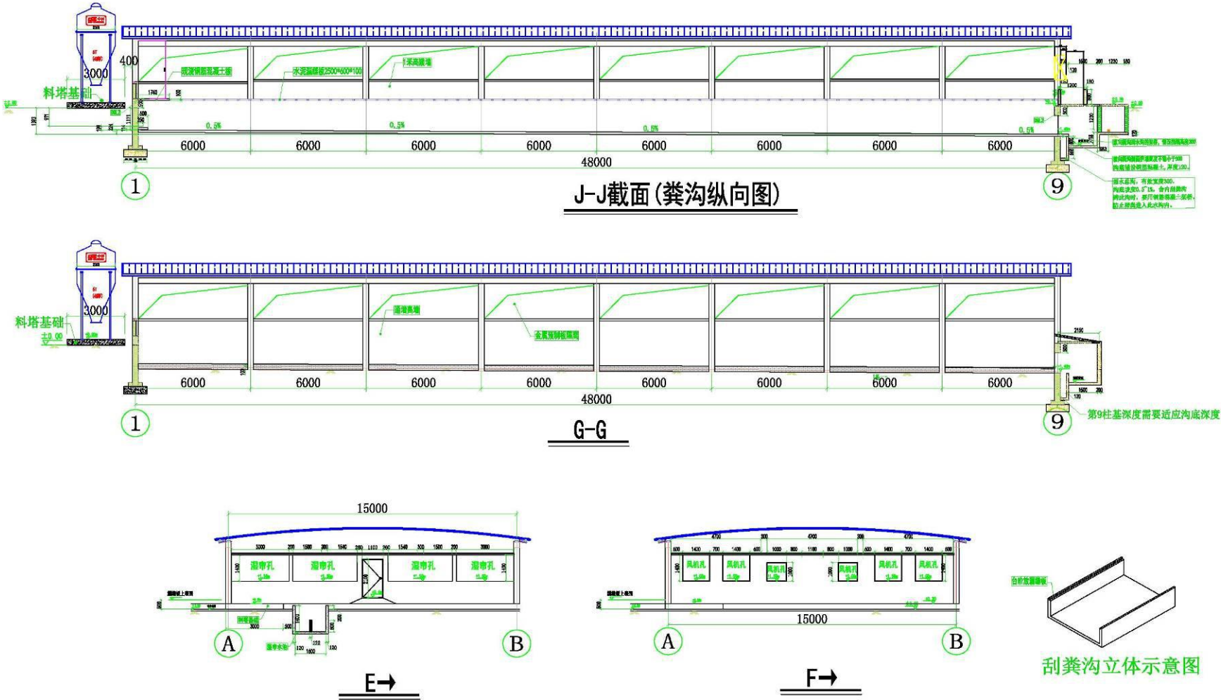
附图 4 粪沟示意图
