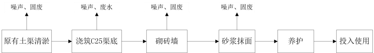
图 5-3 排洪渠改造工艺流程
