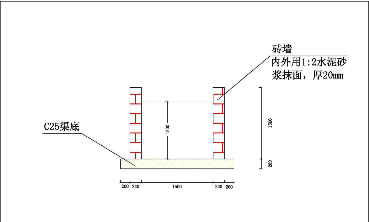
图 1-6 排洪渠改造断面示意图
