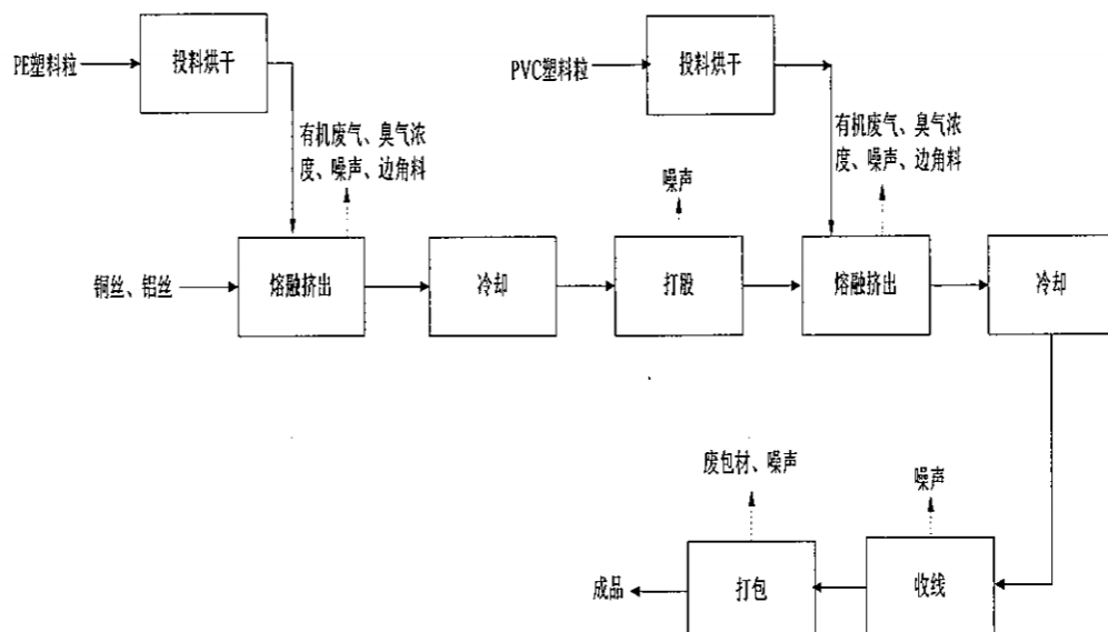
图 2-3 网络线生产工艺流程及产污节点图
