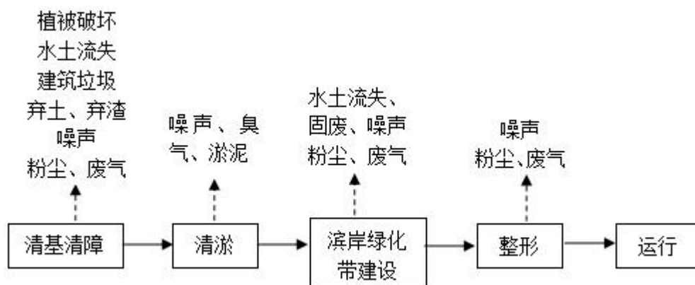
图 2 项目河道清淤工程流程图
