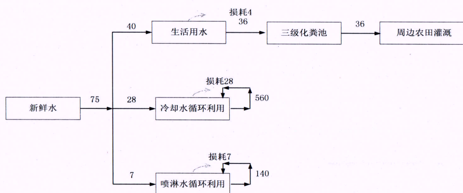
图 2-1 项目用水平衡示意图 (单位: \text{t/a} )
