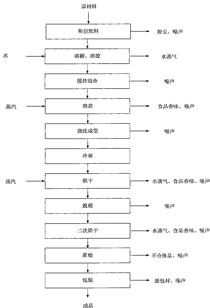
图 2-2 软糖工艺流程图
