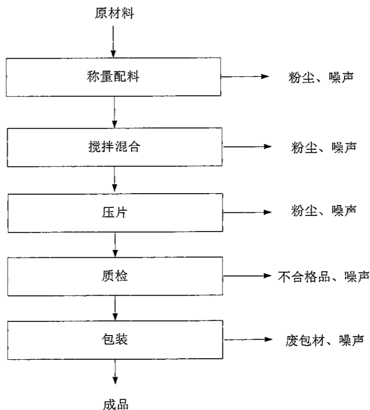
图 2-3 压片糖工艺流程图
