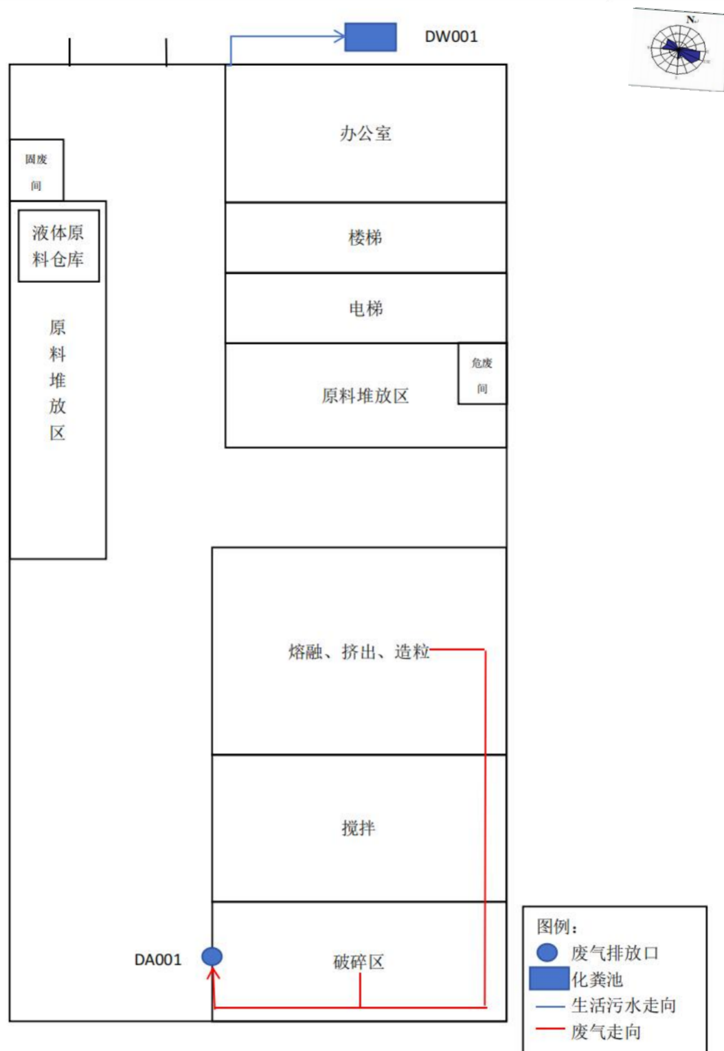
附图 11：平面布局图
