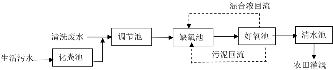
图 7-2 废水处理工艺流程图
