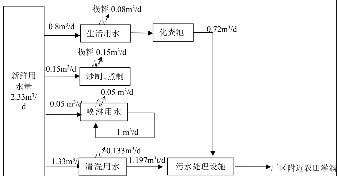
图 5-1 项目水平衡图
