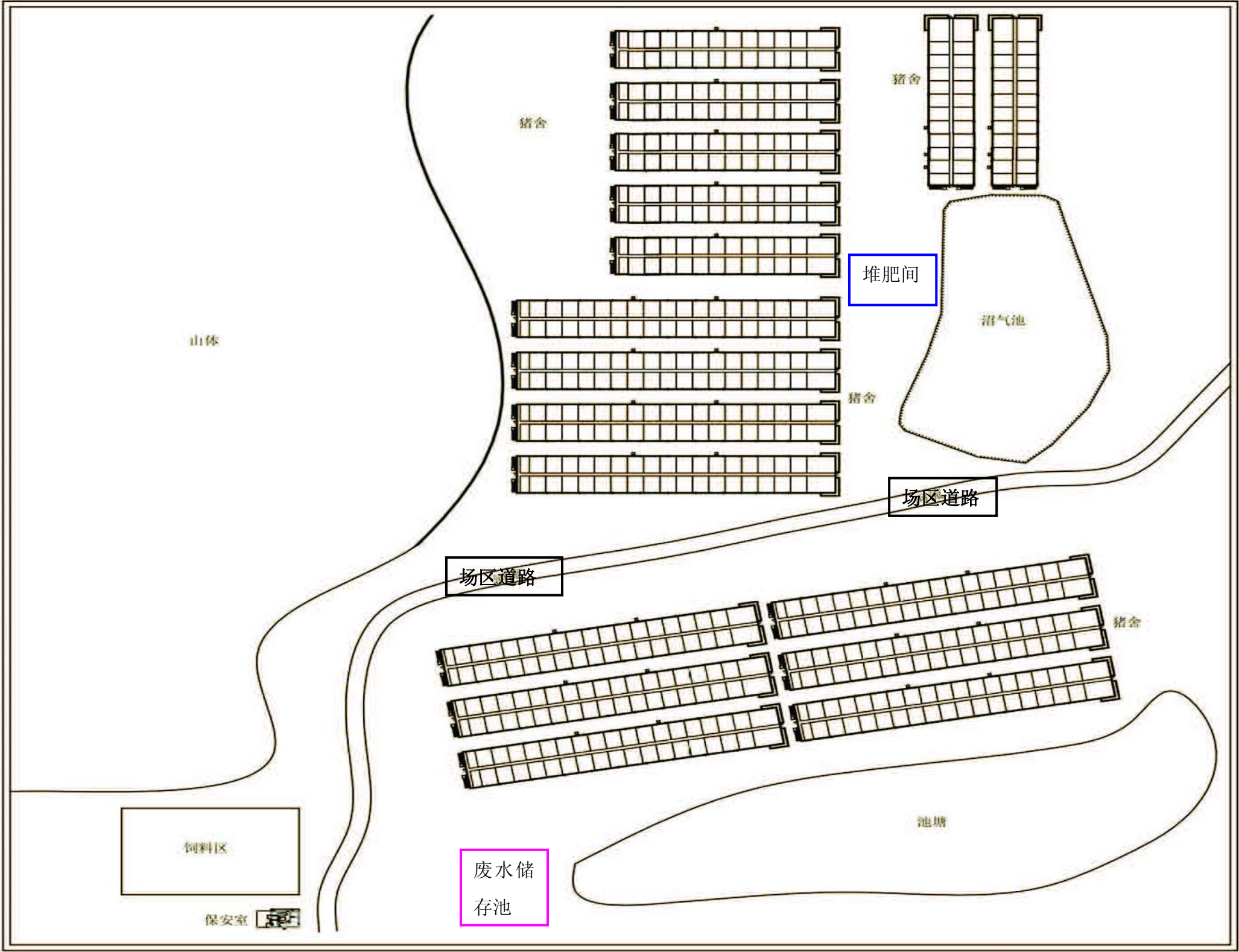
附图 1 项目总平面布置图
