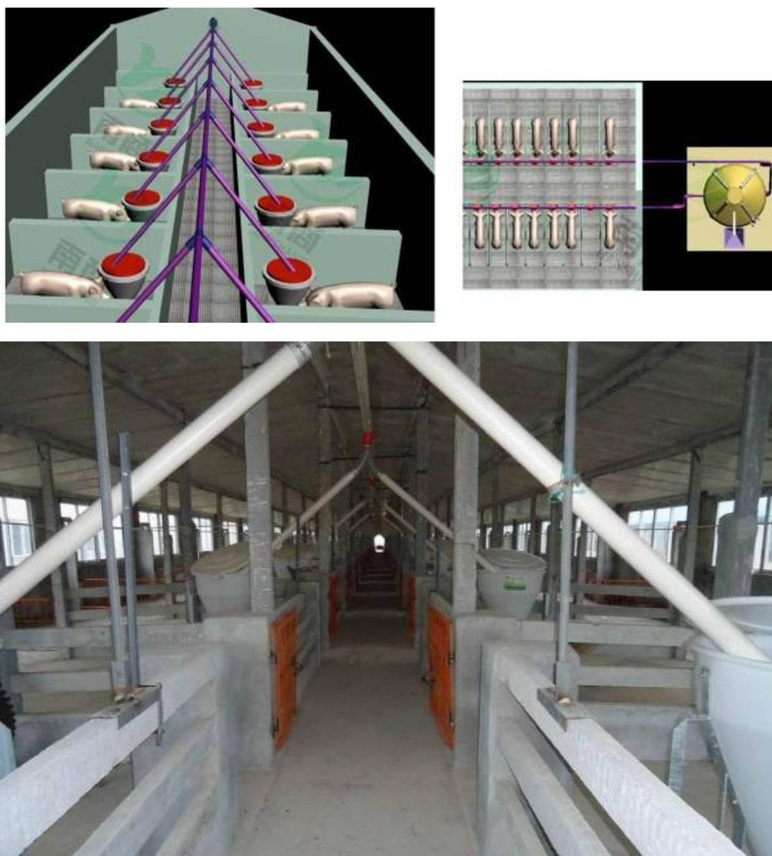
图 2.6-1 自动供料系统
