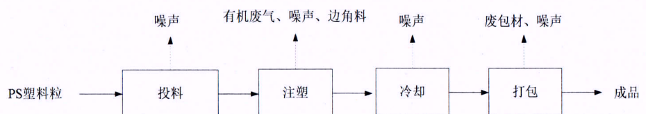
图 2-3 PS 塑料盒工艺流程及产污环节图
