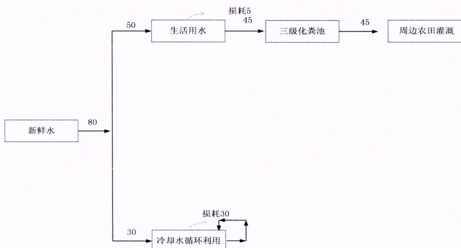
图 2-1 项目水平衡示意图（单位：t/a）
