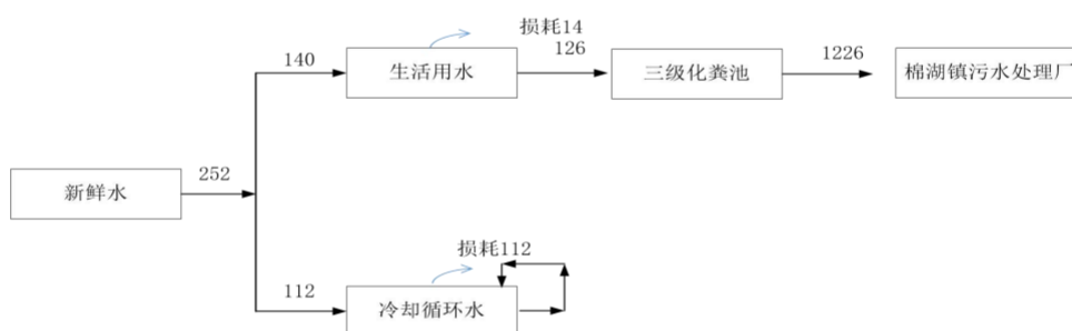
图 2-1 项目用水平衡示意图（单位：t/a）
