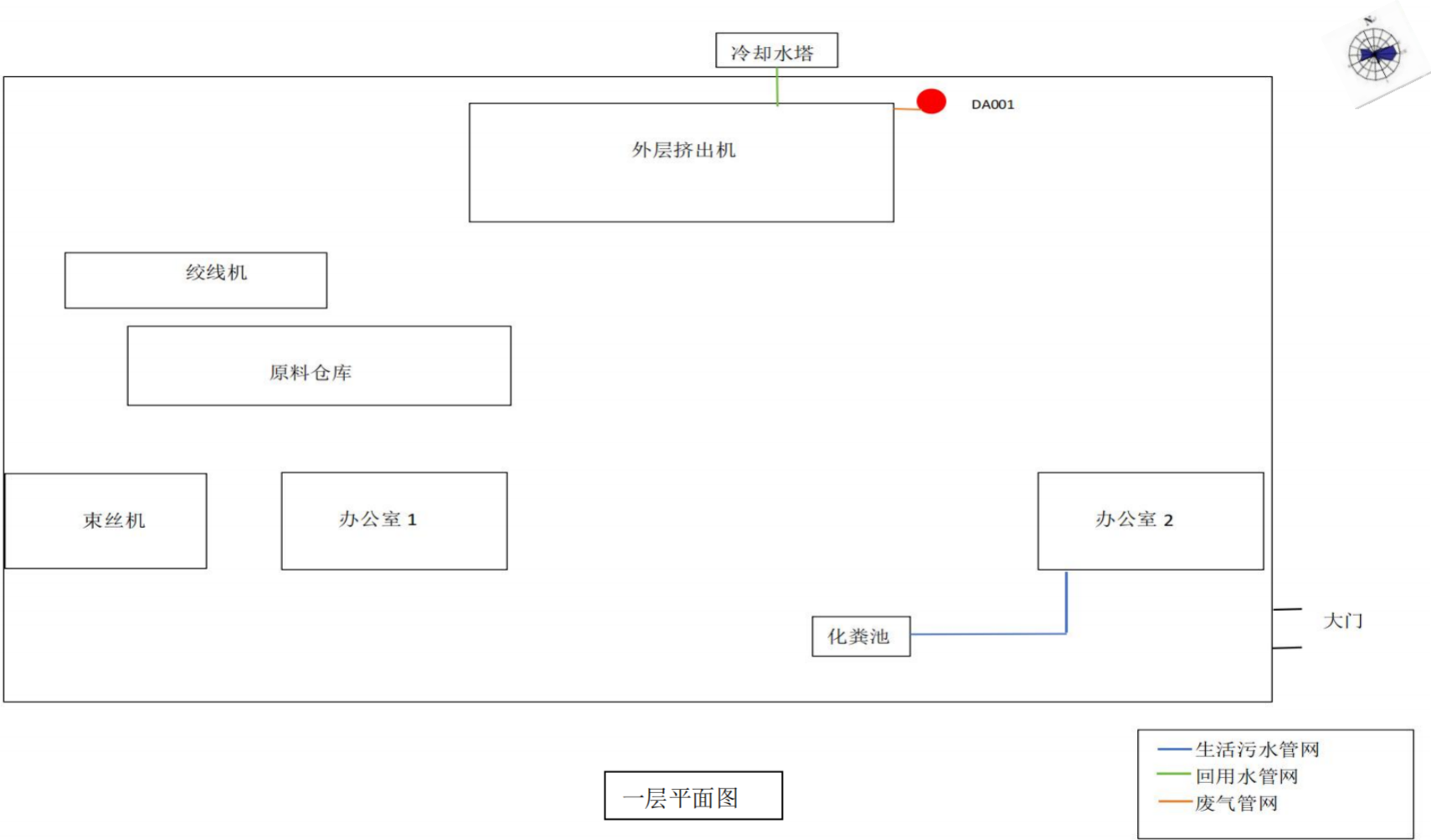
附图 12：平面布局图
