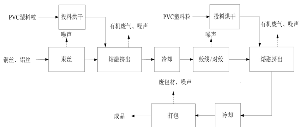
图 2-2 电线生产工艺流程图
