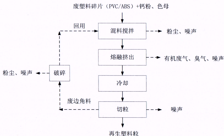
图 2-3 PVC/ABS 再生塑料粒生产工艺流程图
