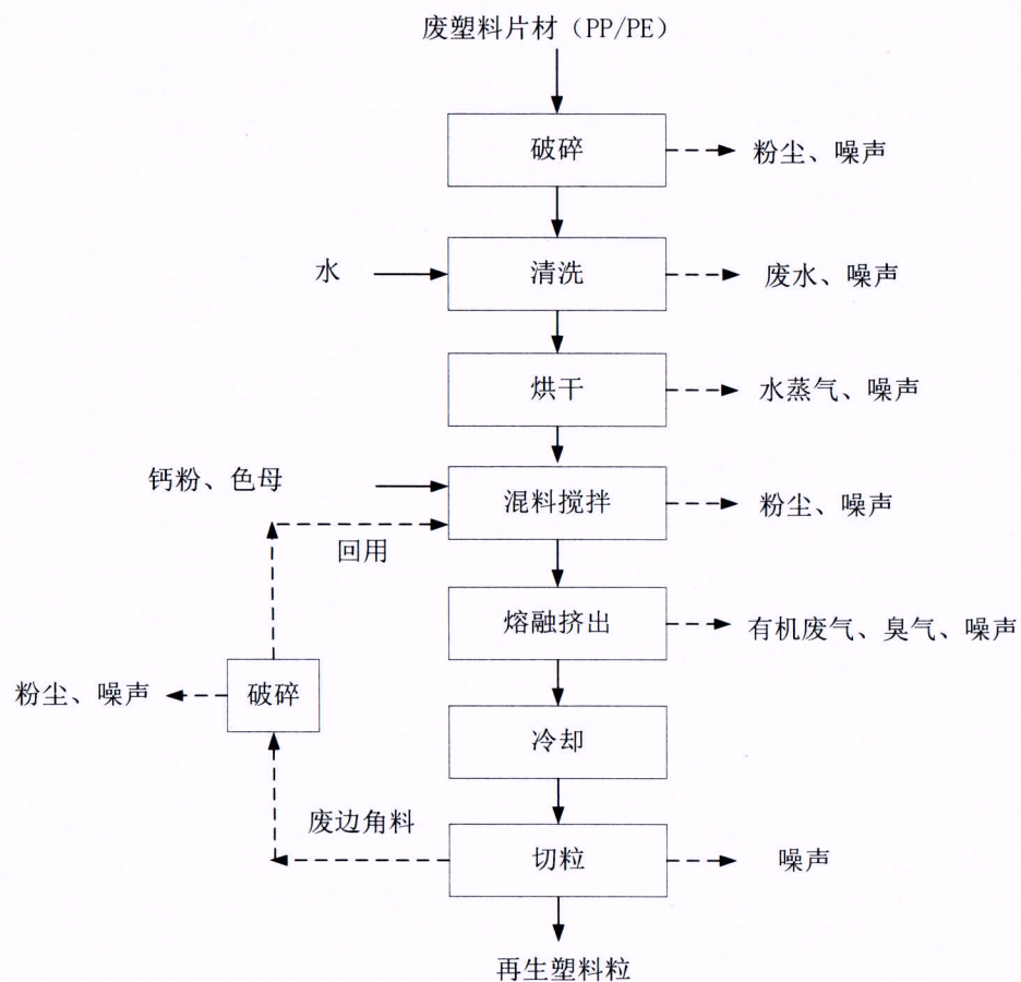
图 2-2 PP/PE 再生塑料粒生产工艺流程图
