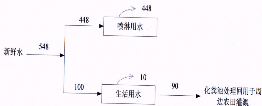
图 2-1 本项目投产后全厂水平衡图 单位： \text{m}^3/\text{a}
