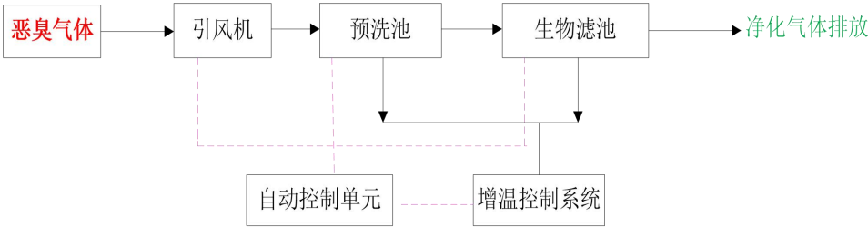
图 4-1 生物滤池除臭工艺流程图
