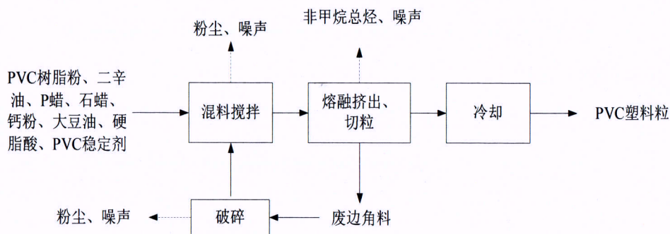
图 2-2 PVC 塑料粒生产工艺流程图
