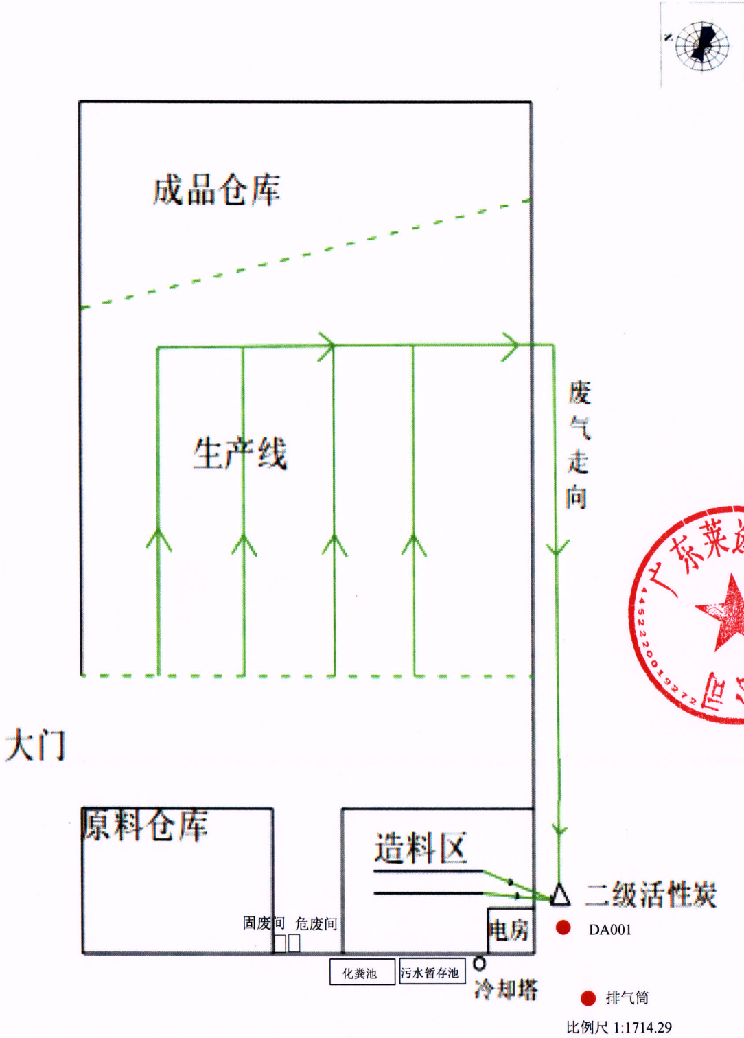
附图 12：平面布局图
