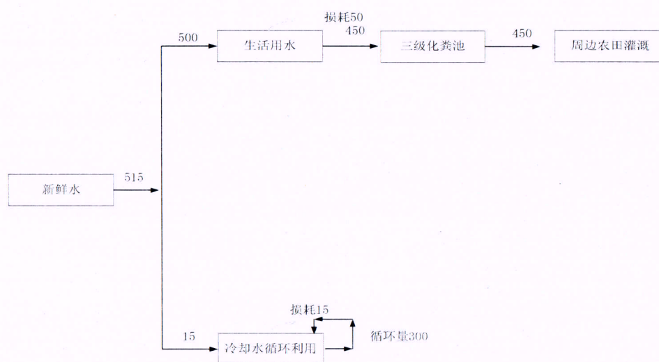
图 2-1 项目用水平衡示意图 (单位: \text{t/a} )
