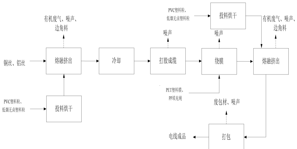
图 2-2 电线生产工艺流程及产污节点图
