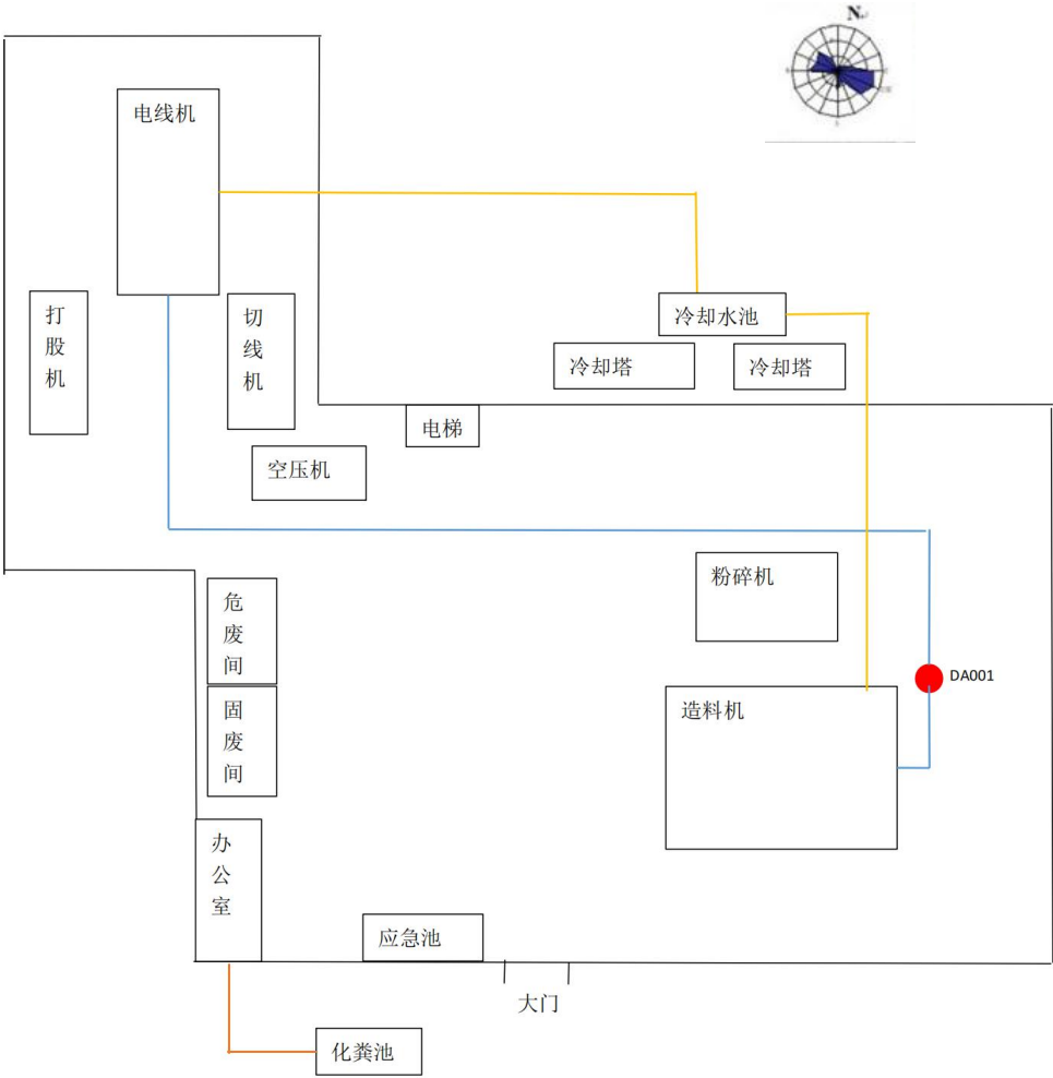
1 楼平面图
