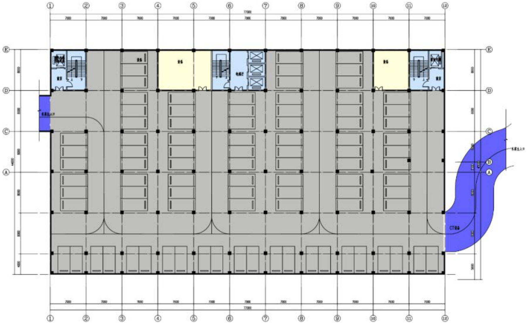
地下室负一平面图 1:100 揭西县棉湖华侨医院住院综合大楼
