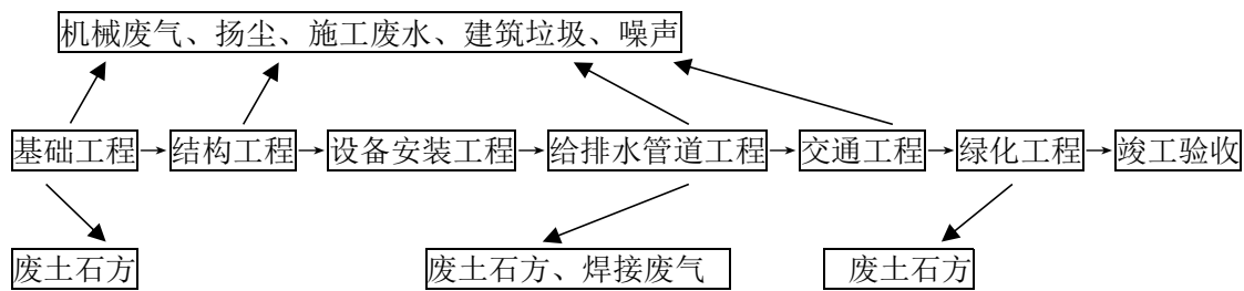
图 5-1 施工期产污工艺流程图
