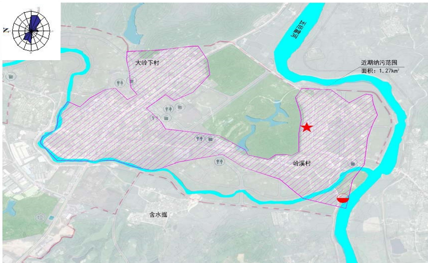
附图 8 京溪园镇污水处理厂服务范围示意图
