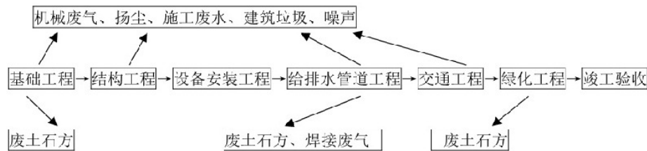
图 5-1 施工期产污工艺流程图
