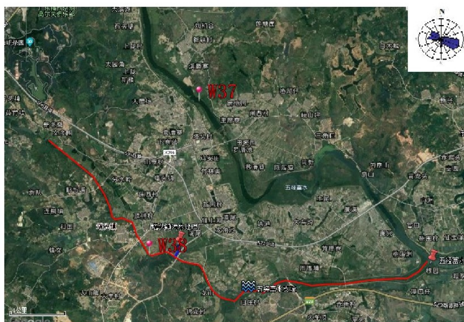
附图 5 水环境监测布点图
